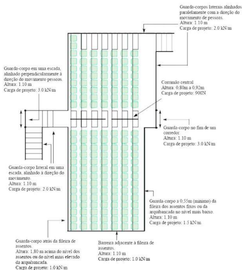
Figura 5 – Barreiras, guarda-corpos e corrimãos centrais: cargas de projeto e altura mínima e disposição.
