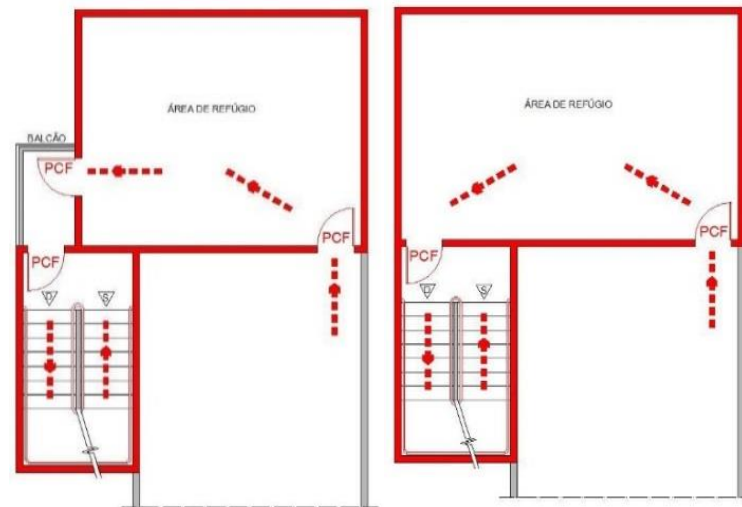
Figura 21 – Desenho esquemático da área de refúgio
