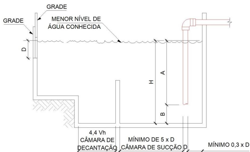
Figura B.5 –Alimentação natural de reservatório por canal
