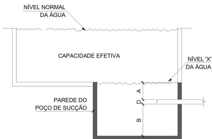
Figura B.1 - Tomada superior de sucção para bomba principal
