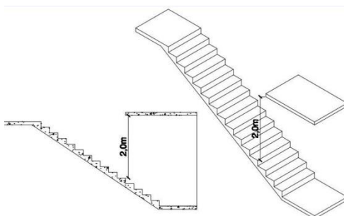
Figura 4 – Altura mínima de pé direito
