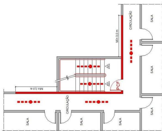
Figura 16 – Escada aberta externa
