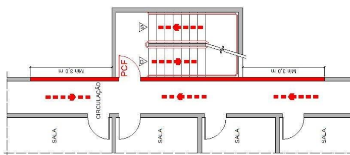
Figura 17 – Escada aberta externa
