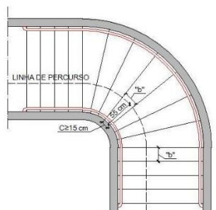
Figura 6 – Escada com lanço misto e degraus balanceados
