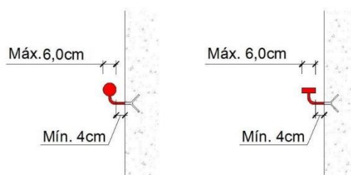
Figura 19 – Pormenores de corrimãos
