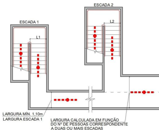
Figura 23 – Dimensionamento de corredores de descarga
