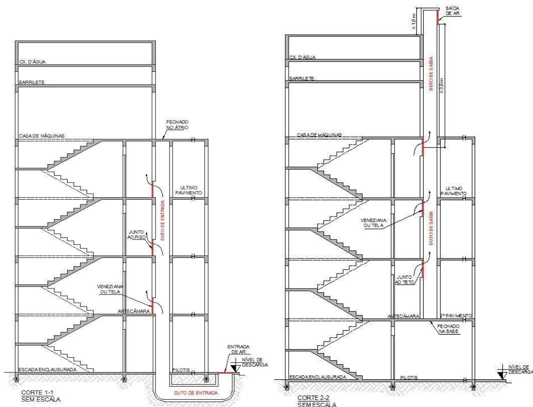
Figura 13 – Antecâmaras e Duto de ar – Desenho esquemático
