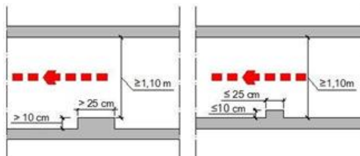
Figura 1 – Medida da largura em corredores e passagens
