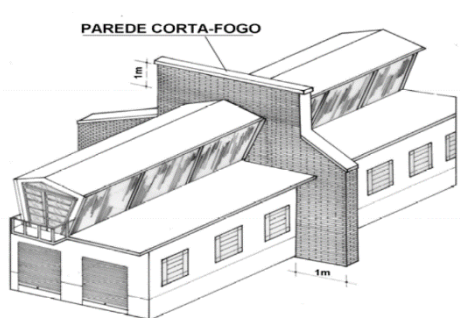
Figura 8 – Parede corta-fogo
